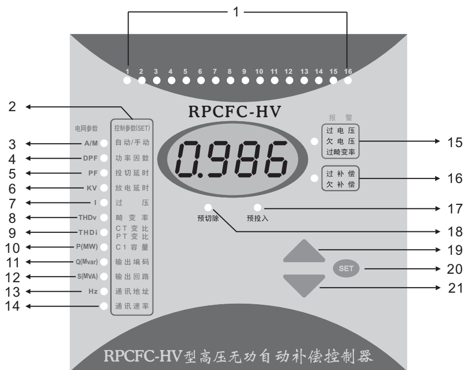
开孔尺寸为140mm×140mm型面板功能图
