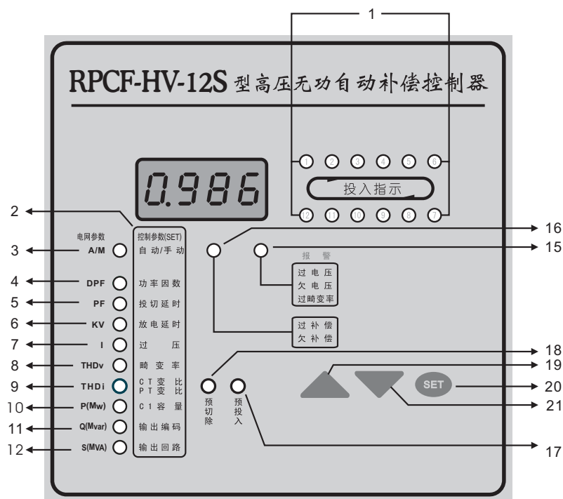
开孔尺寸为113mm×113mm型面板功能图
