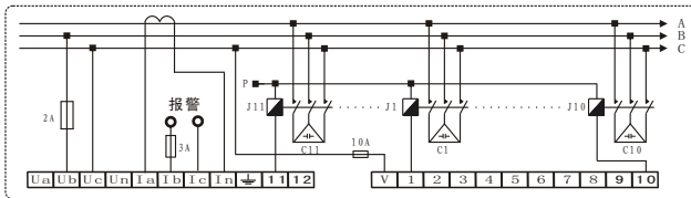
RPC5CM-B-xx型开孔尺寸为113mm×113mm接线图 当交流接触器额定工作电压为380V时P点接B；为220V时接N。
