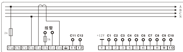
RPC5CS-B-xx型开孔尺寸为113mm×113mm接线图 有源直流电压信号输出输出容量-12V、20mA/路
