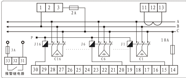
RPC5FM-Bx-xx型开孔尺寸为139mm×139mm接线图 当交流接触器额定工作电压为380V时P点接B；为220V时接N。
