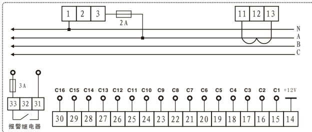
RPC5FS-Bx-xx型开孔尺寸为139mm×139mm接线图 有源直流电压信号输出输出容量-12V、20mA/路
