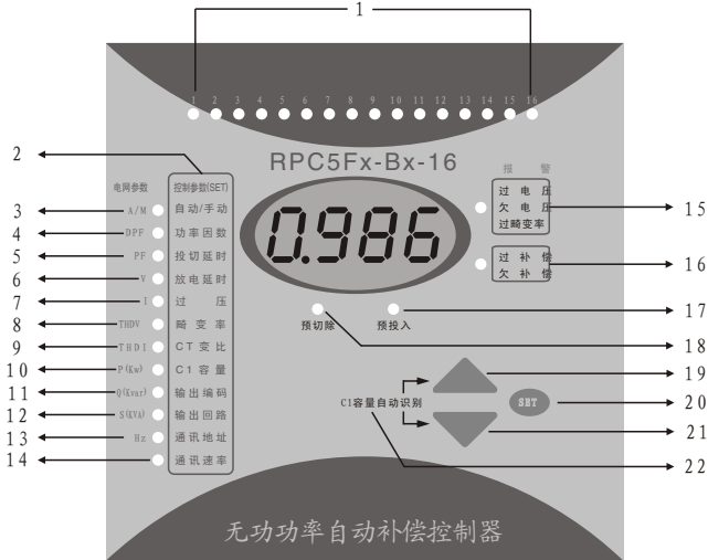
开孔尺寸为139mm×139mm型面板功能图
